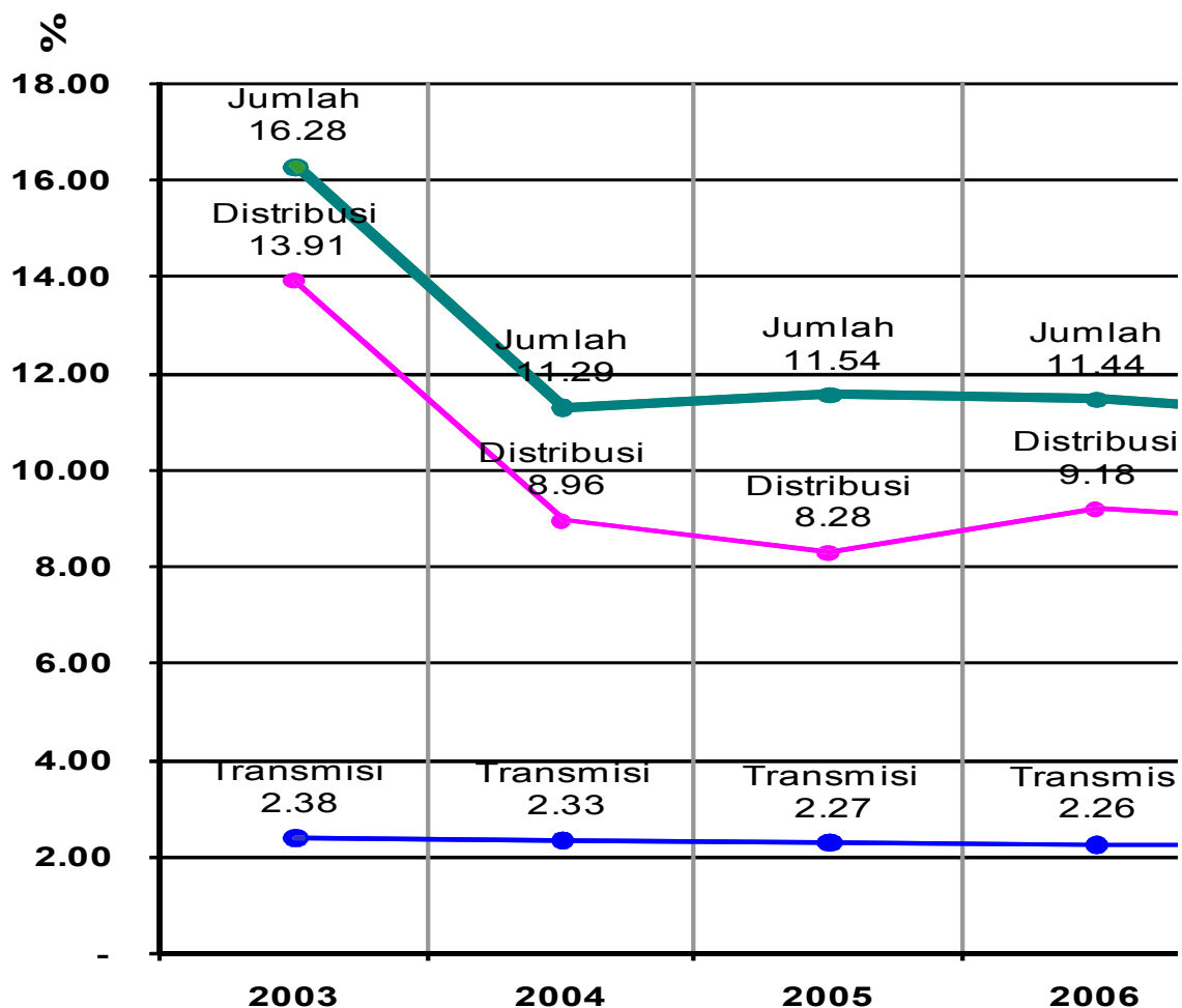
Susut Tenaga Listrik PLN Tahun (20 PLN's Losses Percentage
