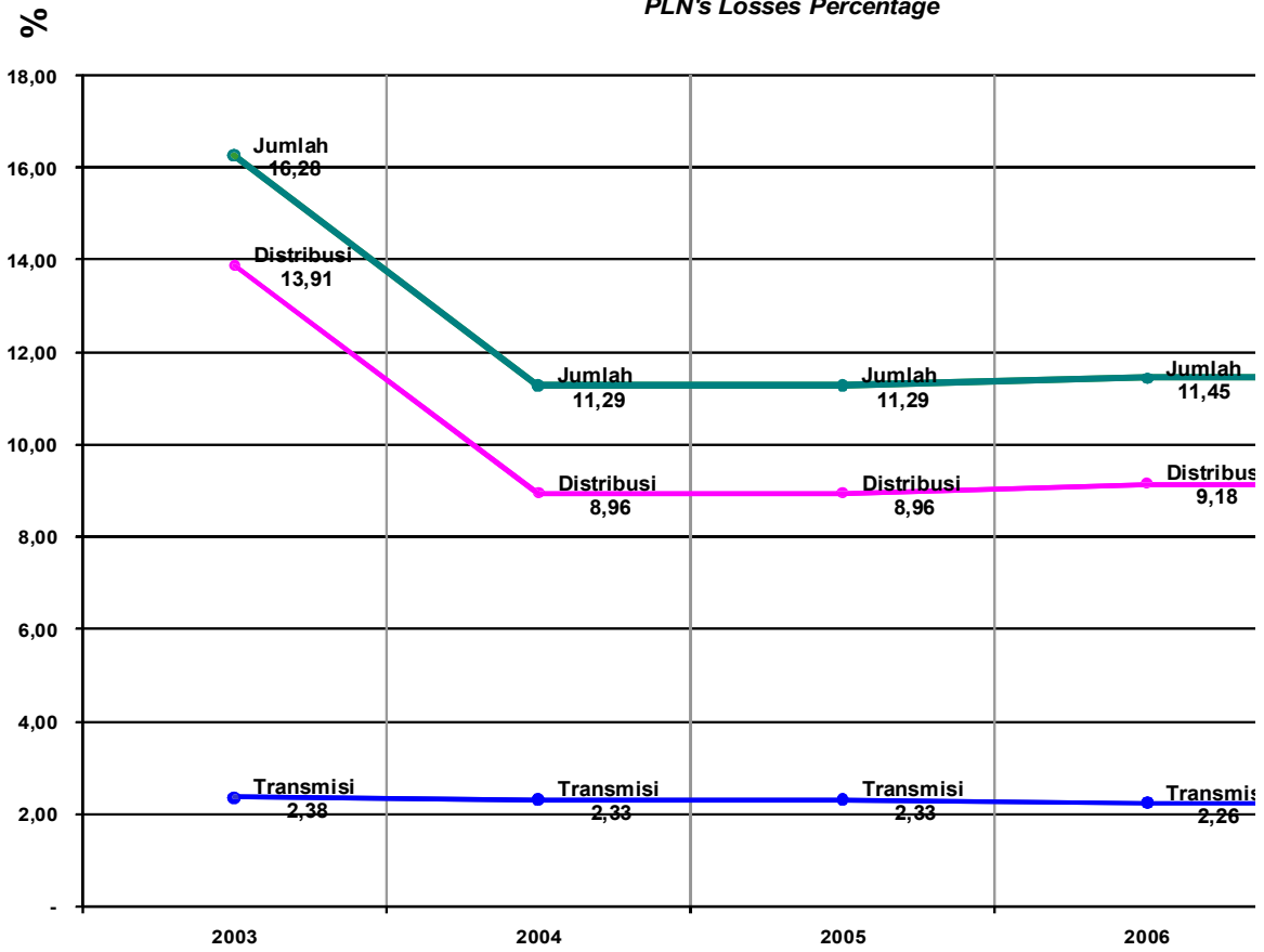
Susut Tenaga Listrik PLN Tahun (2003-2007) PLN's Losses Percentage
