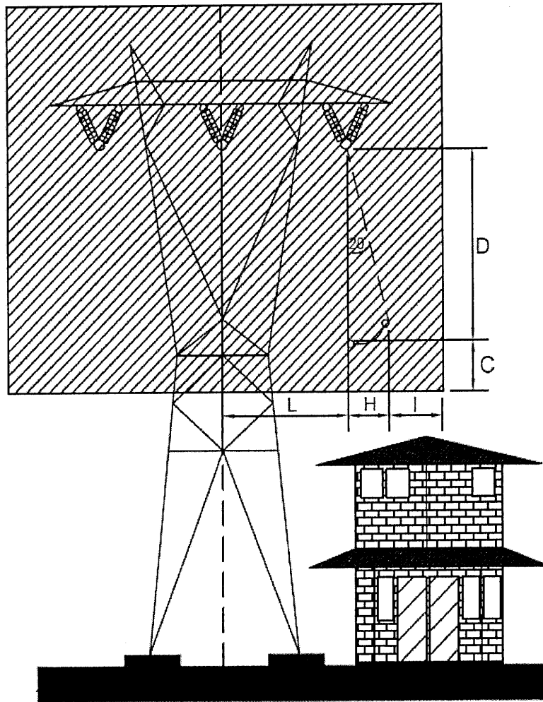
Gambar f. Ruang Bebas SUTET 500 kV Sirkuit Tunggal
