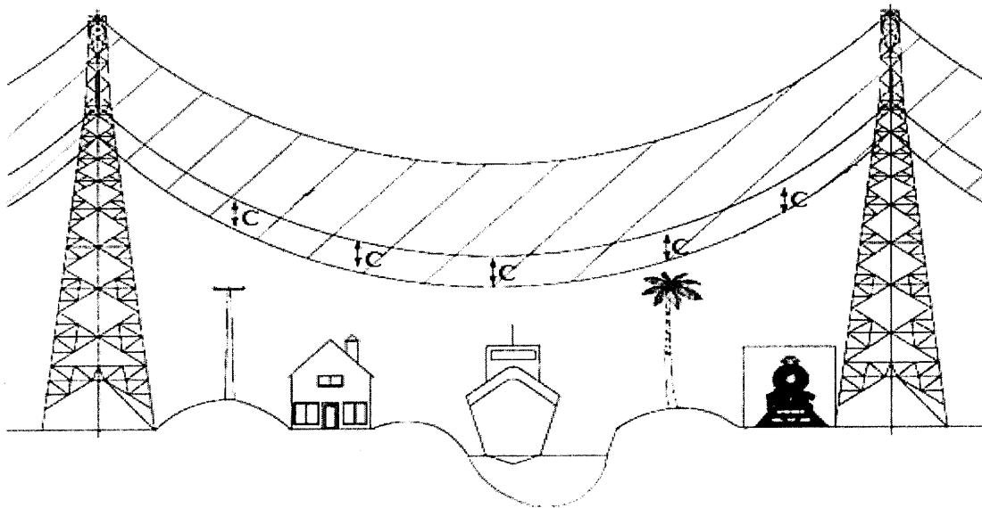
Gambar a. Penampang Memanjang Ruang Bebas
