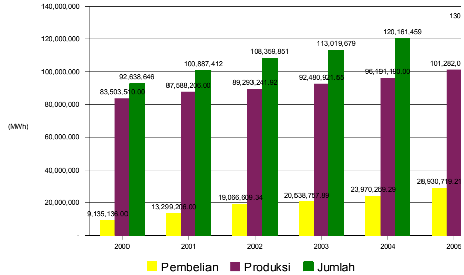
Grafik : Perkembangan Produksi dan Pembelian Tenaga Listrik PLN Tahun 2000 - 2005
