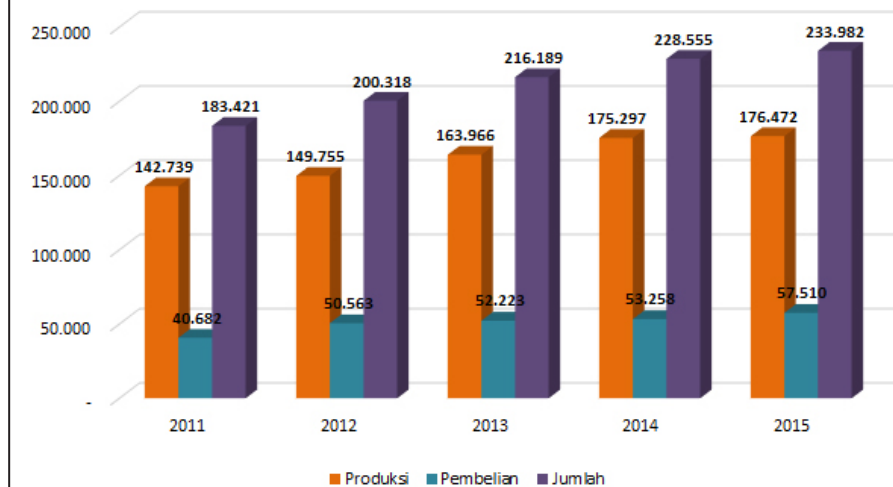
GRAFIK 7 PENYEDIAAN TENAGA LISTRIK PLN TAHUN 2011 - 2015
