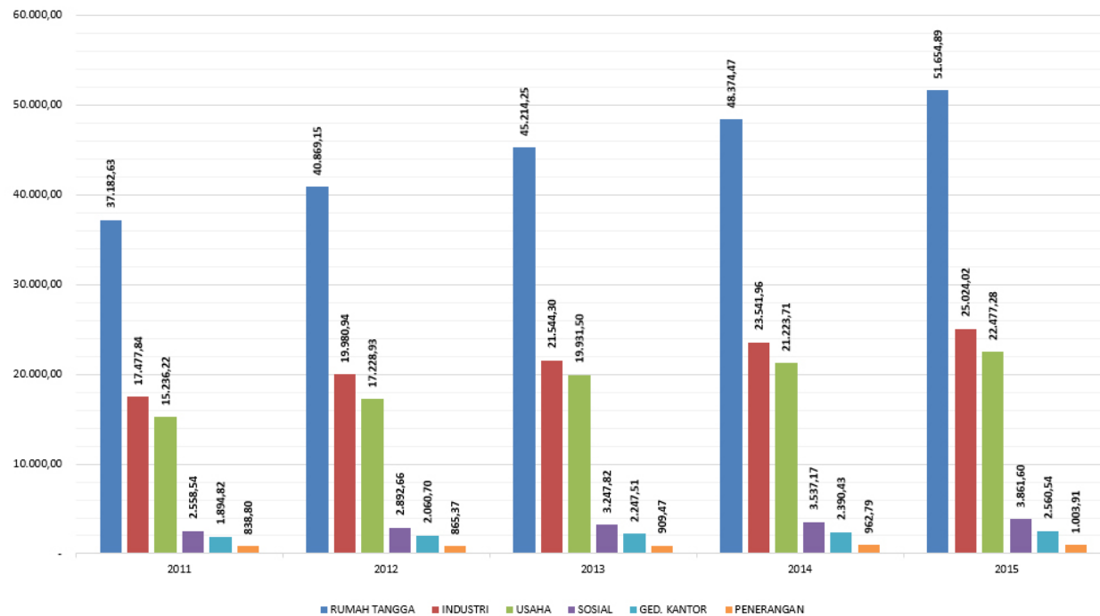
GRAFIK 9 DAYA TERSAMBUNG PER SEKTOR PELANGGAN 2011 - 2015
